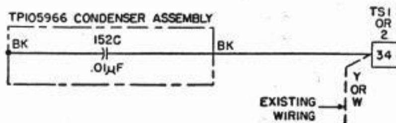
Fig. 3—15A, B and C TTY Bases
