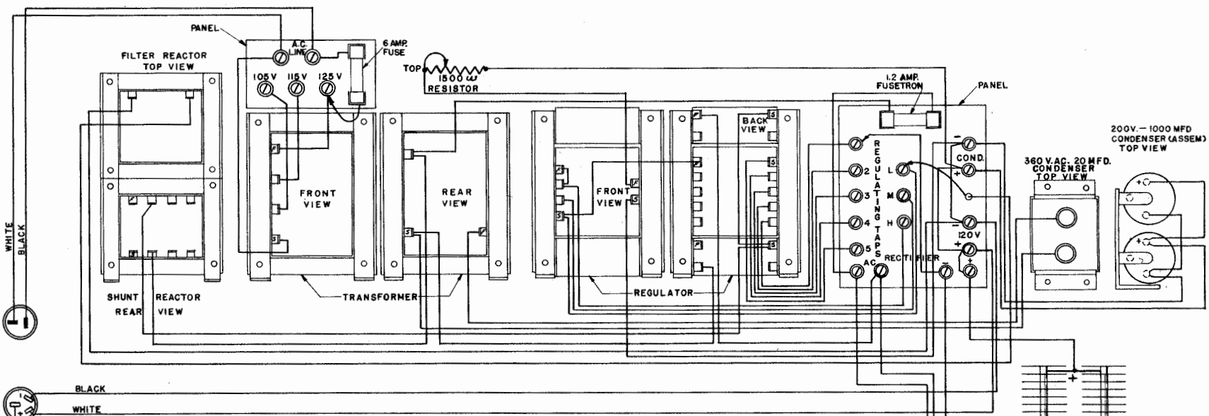
ACTUAL WIRING
