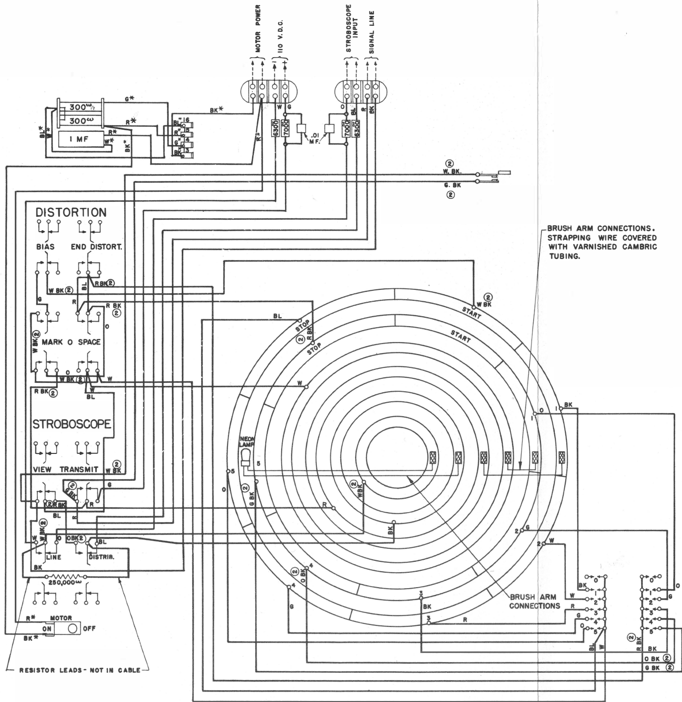
ACTUAL WIRING
