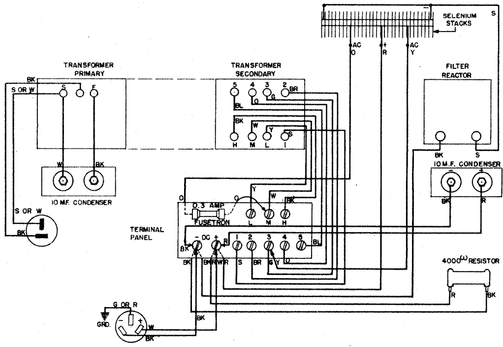
ACTUAL WIRING
