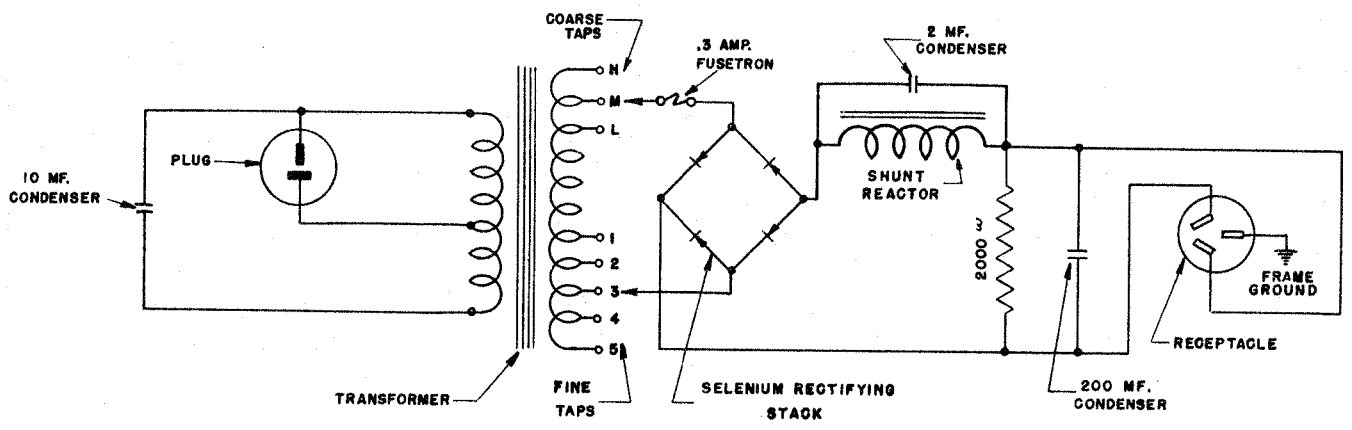
SCHEMATIC WIRING
