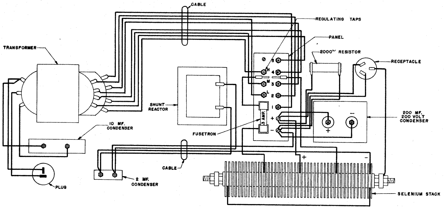
ACTUAL WIRING
