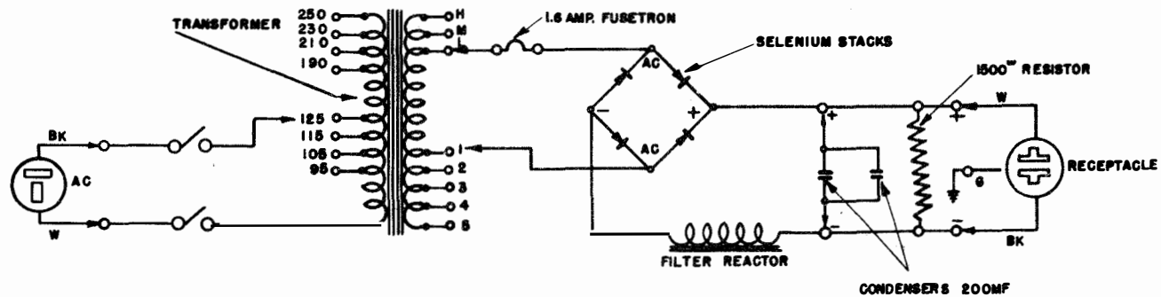
SCHEMATIC WIRING
